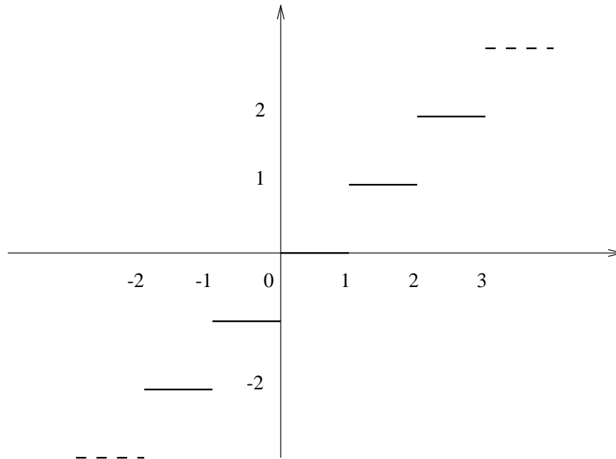
FIGURE 1.1 – graphe de partie entière
